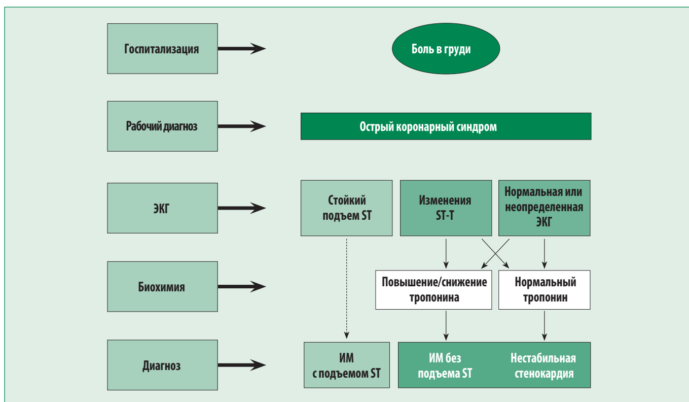
Рис. 1. Спектр ОКС
